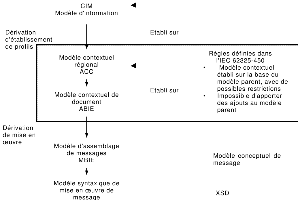
Figure 1 – Cadre de modélisation défini dans l'IEC 62325-450
