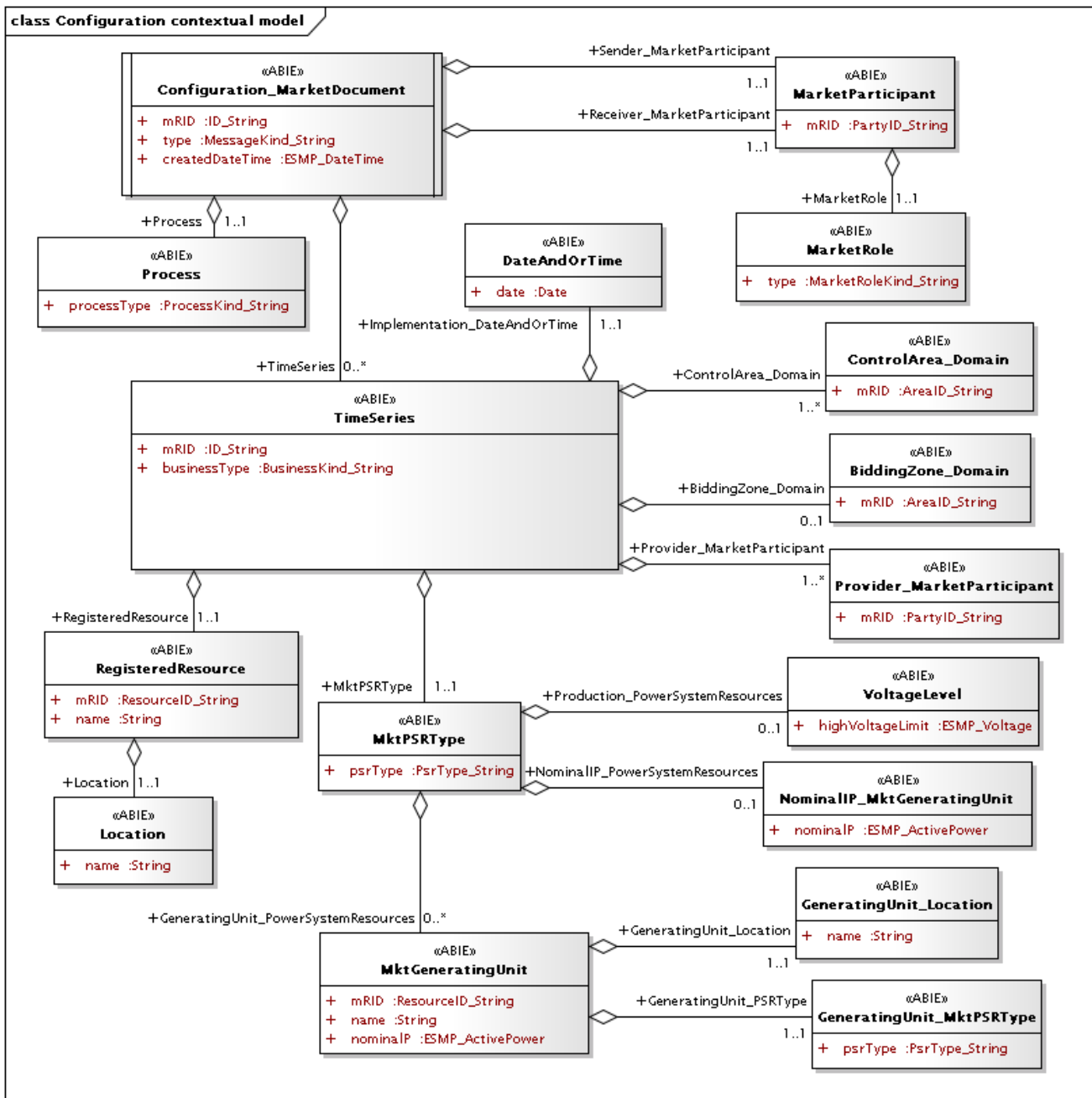
Figure 13 – Modèle contextuel Configuration
