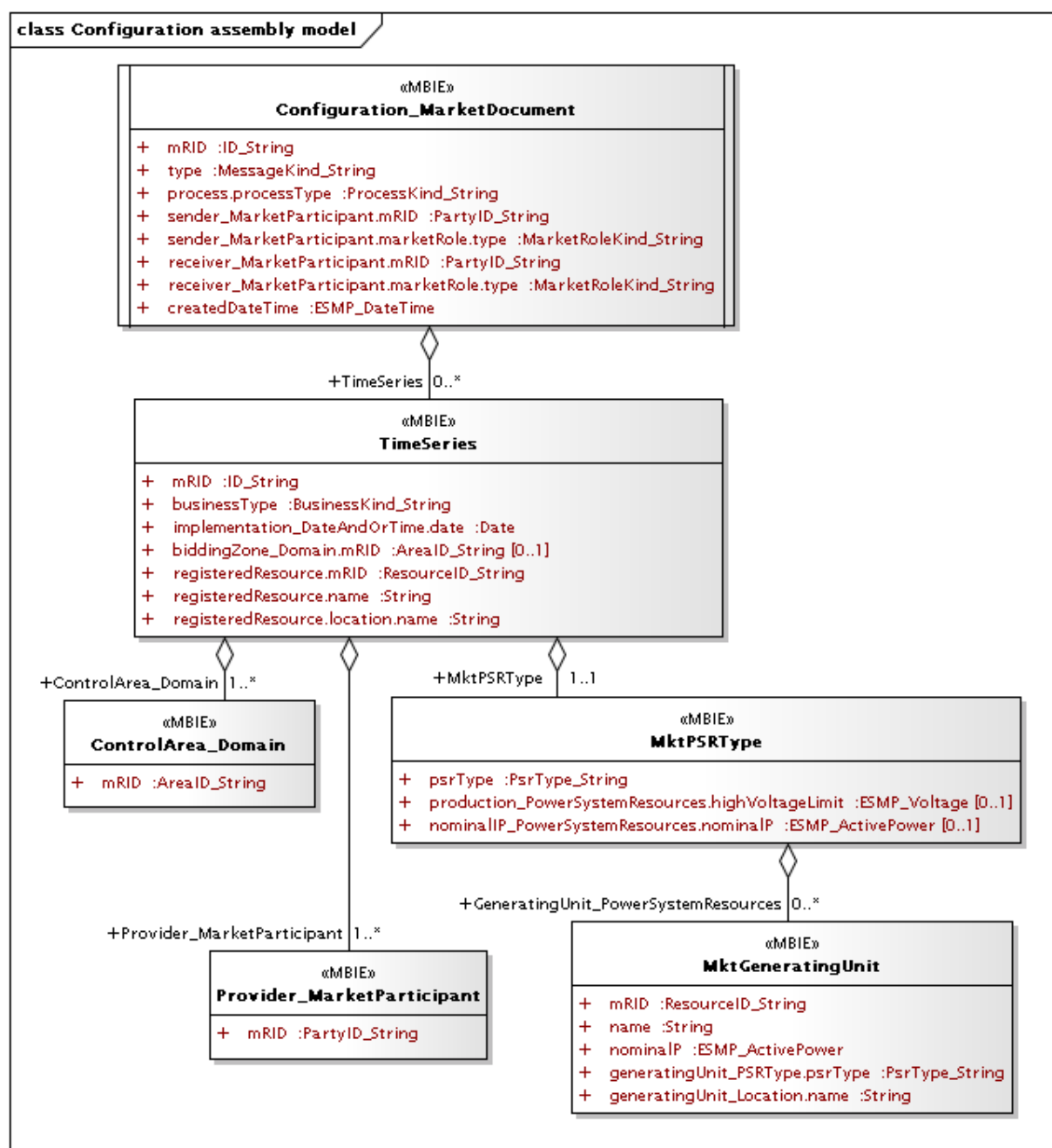
Figure 14 – Modèle d'assemblage Configuration
