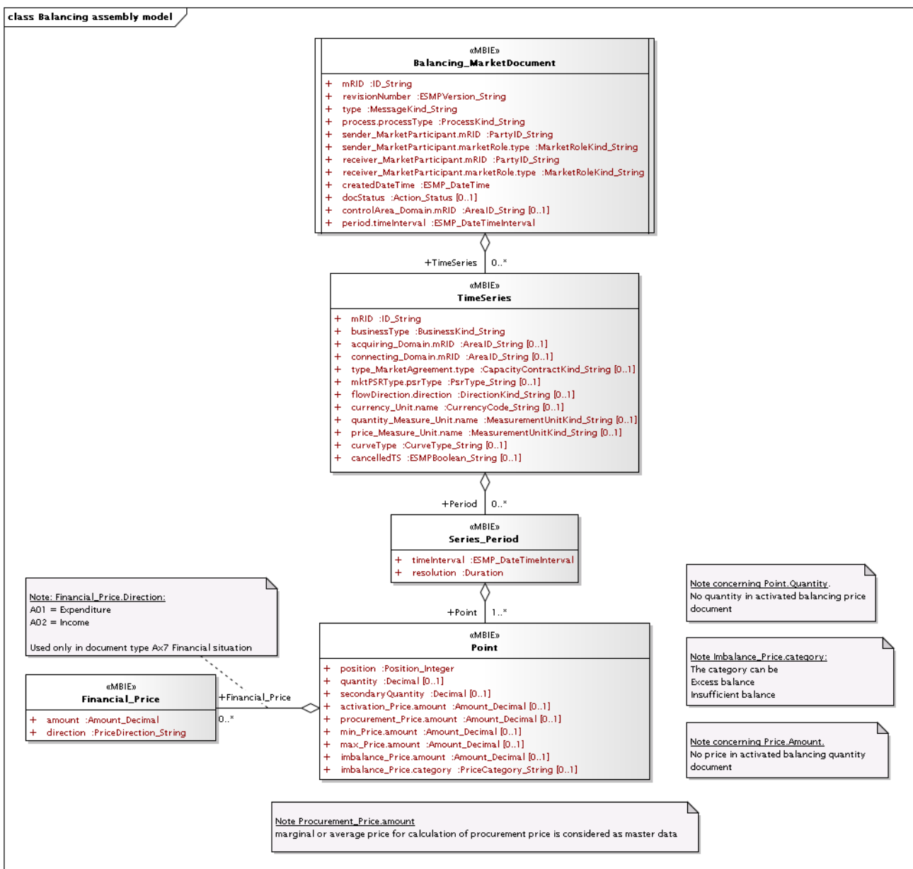
Figure 10 – Modèle d'assemblage Balancing
