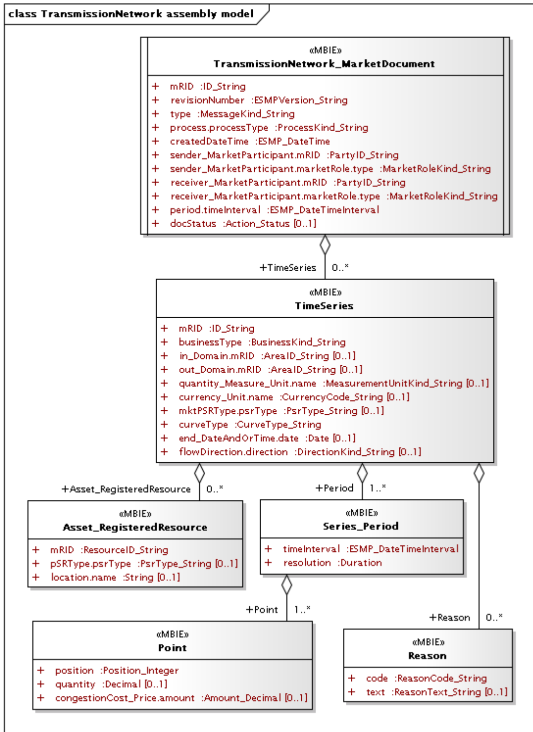
Figure 12 – Modèle d'assemblage TransmissionNetwork
